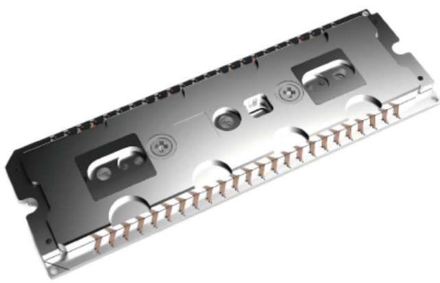
48/32位鱼骨夹具
